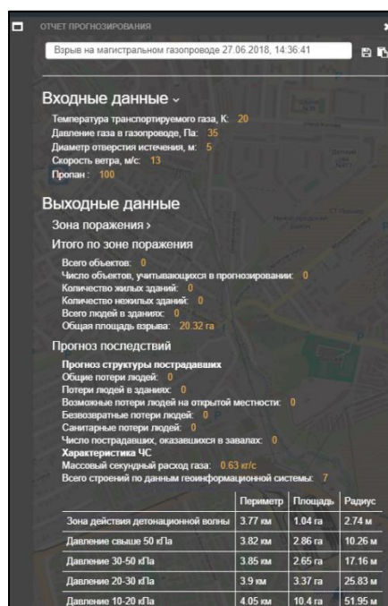
Рисунок 142 — Отчет прогнозирования взрыва на магистральном газопроводе
